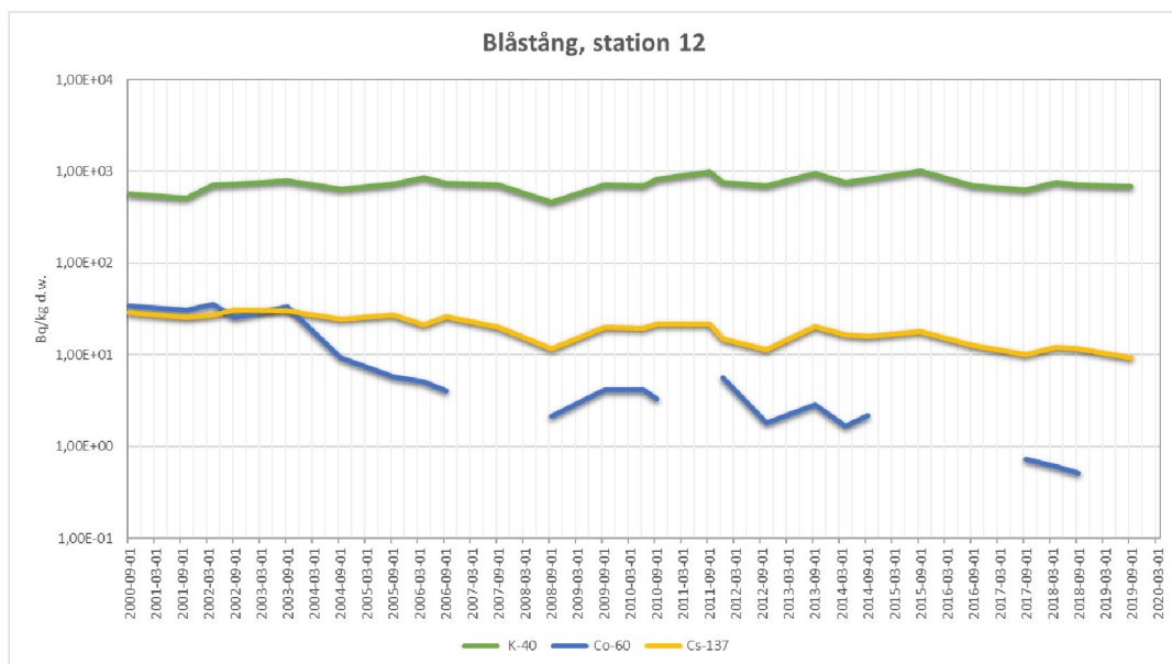
Figur 4. Halten (Bq/kg torrsvikt) av K-40 (grön), Co-60 (blå) och Cs-137 (gul) i blåstång på provtagningsstation 12 utanför OKG och Clab. Co-60 är den av radionukliderna som kan kopplas direkt till driften av anläggningarna på området, medan Cs-137 i huvudsak härrör från Tjernobyl. K-40 förekommer naturligt.
