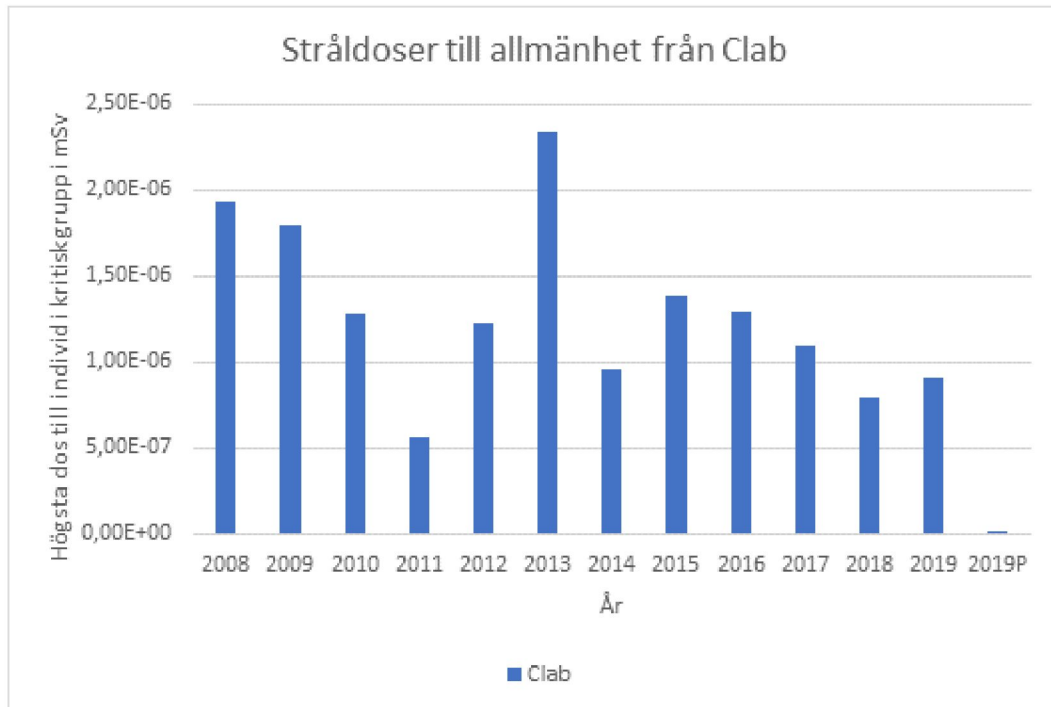
Figur 3 Stråldos till allmänheten från verksamheten vid Clab från 2008 till 2019. Stapeln för 2019P visar dosen beräknad med de nya dosfaktorer enligt PREDO.
