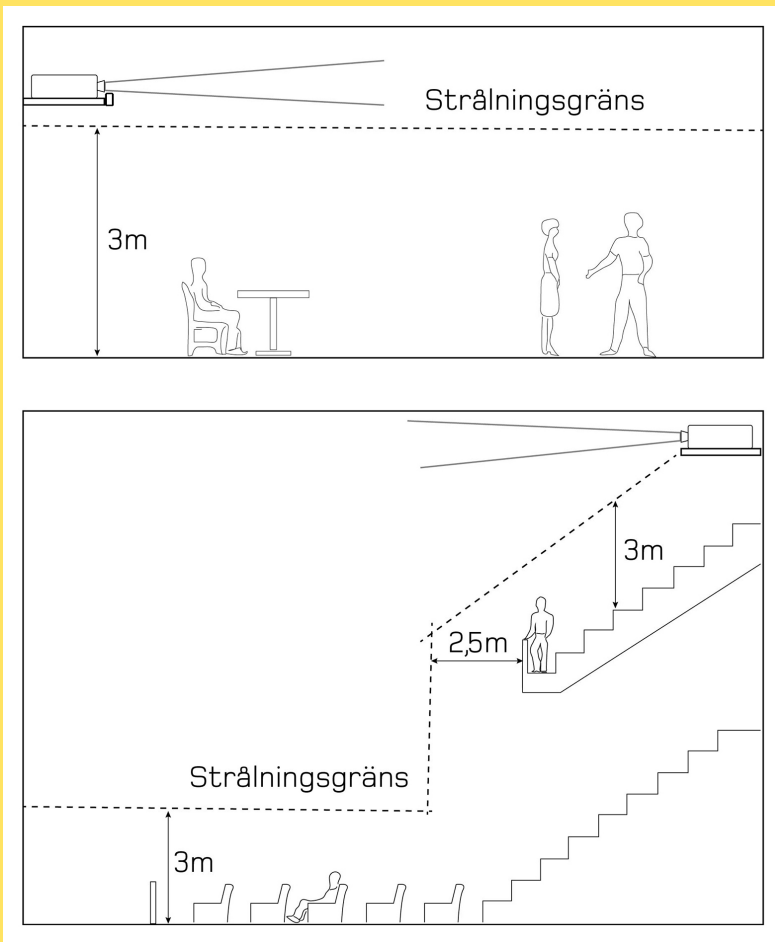
Figur 1: Exempel på begränsningar av strålfältets utbredning annat än i fråga om diffusa reflexer.
