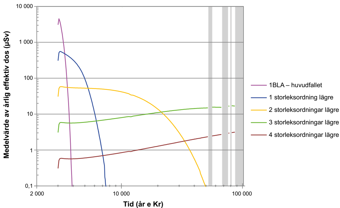
Figur 9-40. Aritmetiskt medelvärde av den årliga dosen för den exponerade gruppen hushåll med köksträdgård för vattenupptag i varianten för intrångsbrunn i 1BLA med alternativa transportegenskaper, där man antar 1 till 4 storleksordningar lägre aktivitetskoncentration i vattnet. Som jämförelse visas även resultatet för beräkningsfallet med intrångsbunnar i 1BLA (ses även i figur 9-39). Vita områden representerar tempererade klimatförhållanden och grå områden periglaciala förhållanden med kontinuerlig permafrost.
