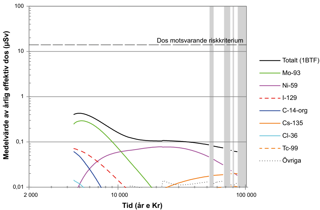
Figur 9-33. Aritmetiskt medelvärde av den årliga dosen till den exponerade gruppen jordbrukare på dikade myrar i biosfärsobjekt 157_2 för utsläpp från 1BTF i scenariot med höga koncentrationer av komplexbildare . Vita områden representerar tempererade klimatförhållanden och grå områden periglaciala förhållanden med kontinuerlig permafrost.
