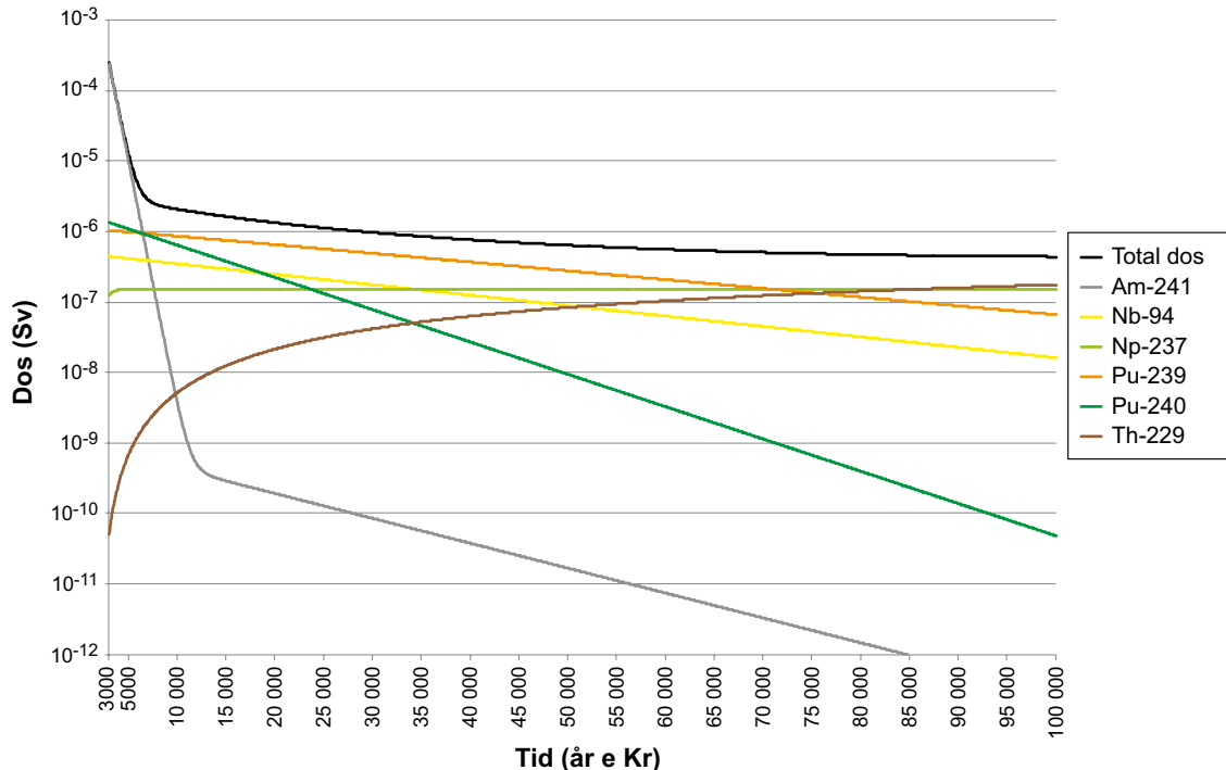
Figur 9-41. Dosen i FHA-scenariot borrar i förvaret vid exponering av personal på plats under borrar, för rotationsborrning med luft i silon (från FHA-rapporten figur 5-2a).
