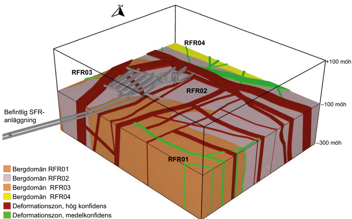
Figur 4-40. Bergdomäner och deformationszoner i SFR:s lokala modell, version 1.0 betraktad snett nedåt mot norr. Blockets läge visas i figur 4-39 (SKB 2013e, figur 5-2).
