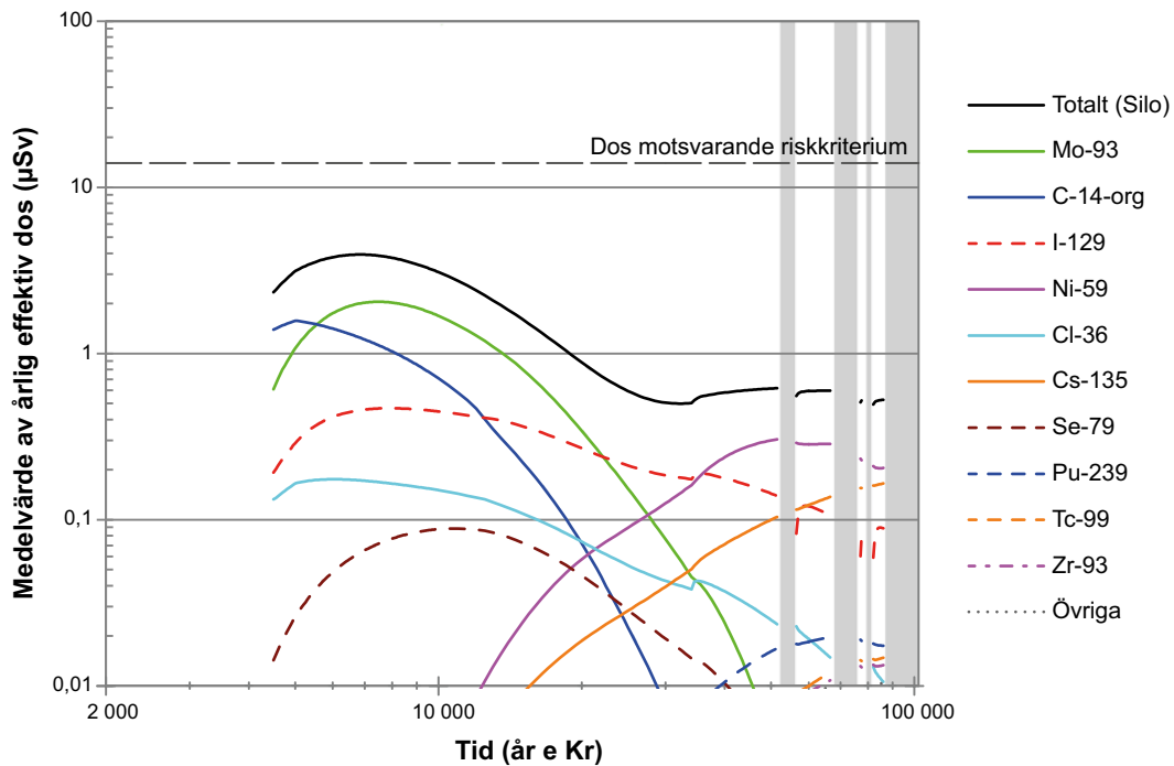
Figur 9-23. Aritmetiskt medelvärde av den årliga dosen till den exponerade gruppen jordbrukare på dikade myrar i biosfärsobjekt 157_2 för utsläpp från silon i scenariot med accelererad betongdegradering. Vita områden representerar tempererade klimatförhållanden och grå områden periglaciala förhållanden med kontinuerlig permafrost.
