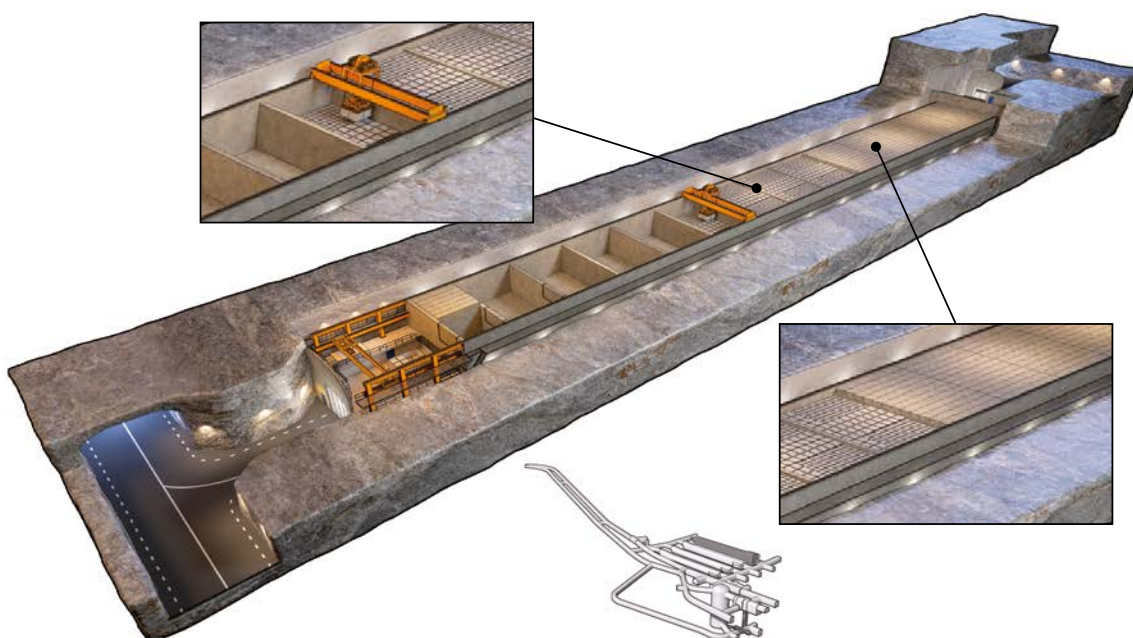
Figur 4-5. Bergssal för medelaktivt avfall, 1BMA, i SFR 1 under driftskedet.
