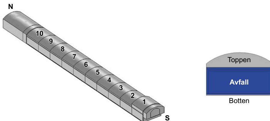
Figur 8-9. Sektioner (till vänster) och kontrollvolymer (till höger) för den hydrologiska modellen för 1-2BTF (Abarca et al. 2013).
